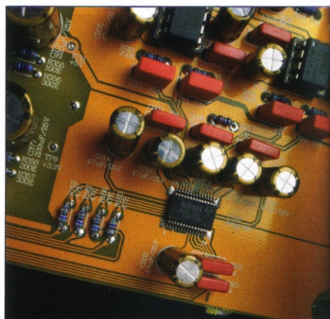
Der D/A-Wandler kann per Upsampling mit bis 192 kHz/24 Bit angefahren werden
